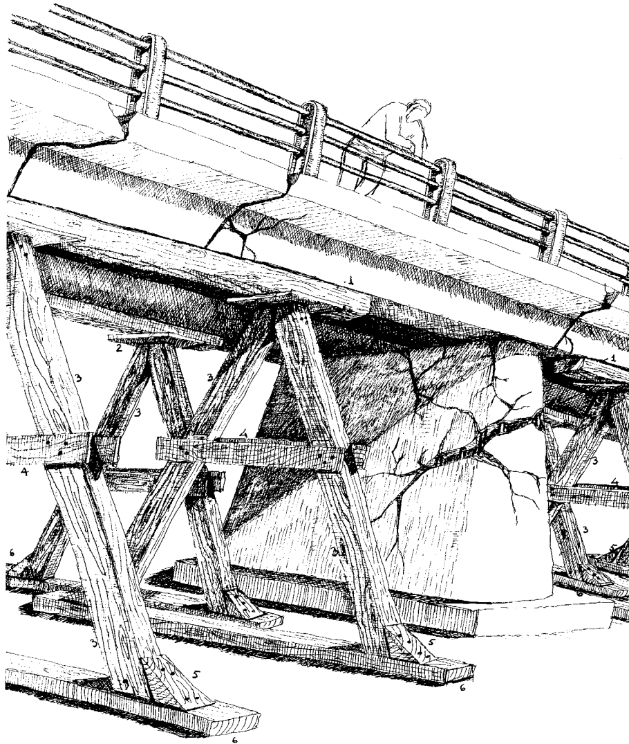
Σχ. 5. Πολλαπλή τριγωνική υποστήλωση με ξύλινες δοκούς εκατέρωθεν βλαμμένου βάθρου γέφυρας
