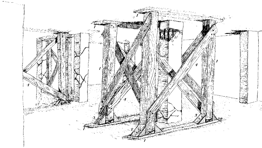
Σχ. 4.α 1 Υποστύλωση με ξύλινους στύλους γύρω από βλαμμένο υποστύλωμα 1. Ορθοστάτες 2. Σανίδαμα στήριξης 3. Σφήνες τριγωνικές 4. Χιαστί σύνδεσμοι μπρος - πίσω
