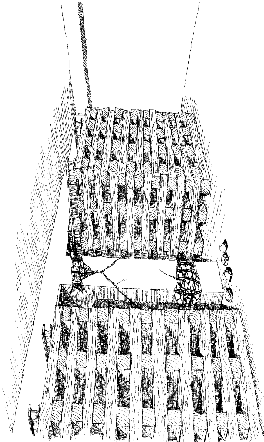
Σχ. 7. Ισχυρή υποστήλωση με τακτορία εκατέρωθεν βλαμμένου υποστυλώματος
