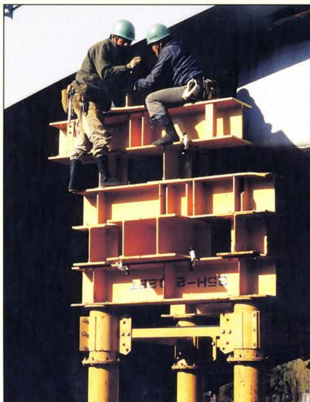
ΚΟΜΠΕ Ιαπωνίας 1995 Εκτεταμένες και βαρείες υποστυλώ- σεις με «πάσης φύσεως» σιδηρές δια- τομές, βαρέως τύπου σε μεγάλες γέφυρες της πόλης, που υπέστησαν σοβαρές βλάβες στα βάθρα τους και σε μήκος πολλών χιλιομέτρων.
