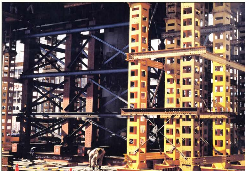
ΚΟΜΠΕ Ιαπωνίας 1995 Εκτεταμένες και βαρείες υποστυλώ- σεις με «πάσης φύσεως» σιδηρές δια- τομές, βαρέως τύπου σε μεγάλες γέφυρες της πόλης, που υπέστησαν σοβαρές βλάβες στα βάθρα τους και σε μήκος πολλών χιλιομέτρων.
