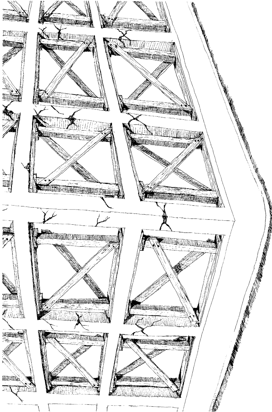
Σχ. 11. Αντιστήριξη με διαγώνιους συνδέσμους και δημιουργία πλαίστιων ακρίματος Π (σε πολλές αράφους)
