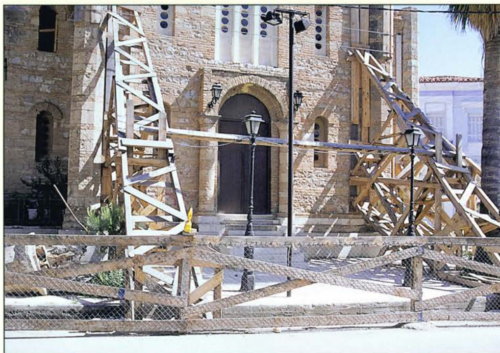
ΑΙΓΙΟ 1995 Εκτεταμένη αντιστήριξη με βιομηχανική ξυλεία στο Ναό Εισοδίων της Θεοτόκου - Έργο Ταϊλλερ, - ο οποίος υπέστη σοβαρές βλάβες.
