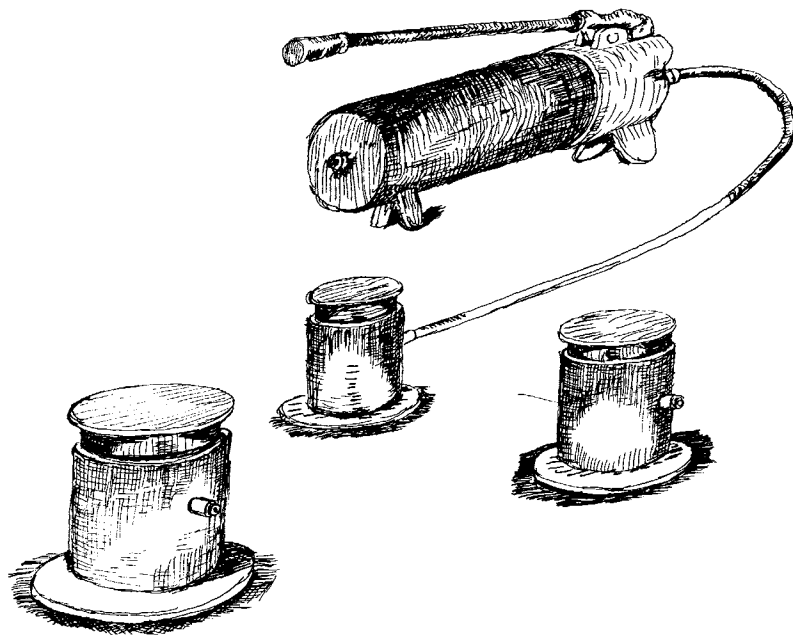
Σχ. 17. Μηχανικοί – υδραυλικοί γρύλοι
