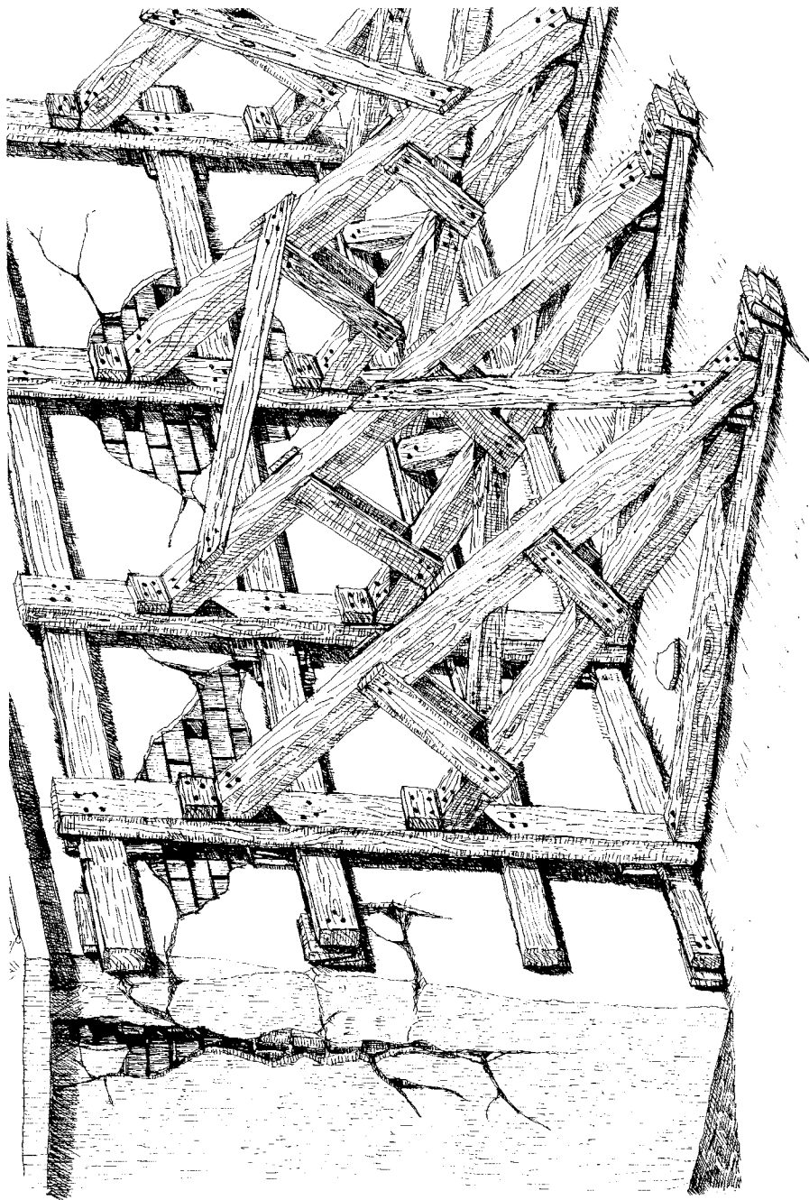
Σχ. 10. Λοξή αντιστήριξη τοίχου με ξύλινες αντηρίδες
