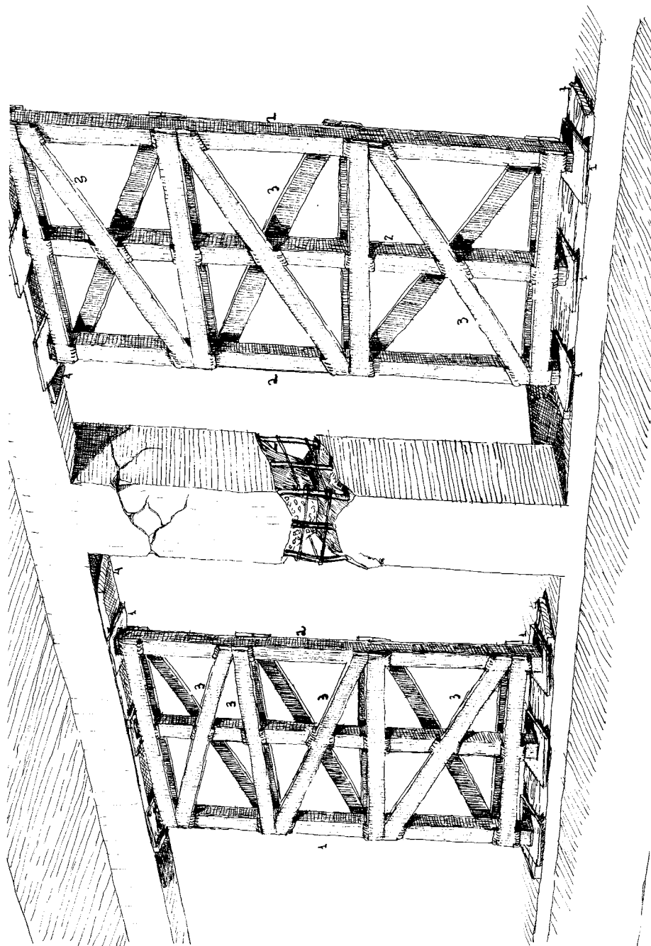
Σχ. 3.δ Υποσύστημα με κοιλοδοκούς εκατέρωθεν "σπασμένου" υποστυλώματος
